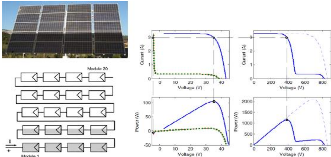
Figure 55 - Ombrage partiel sur une chaîne
